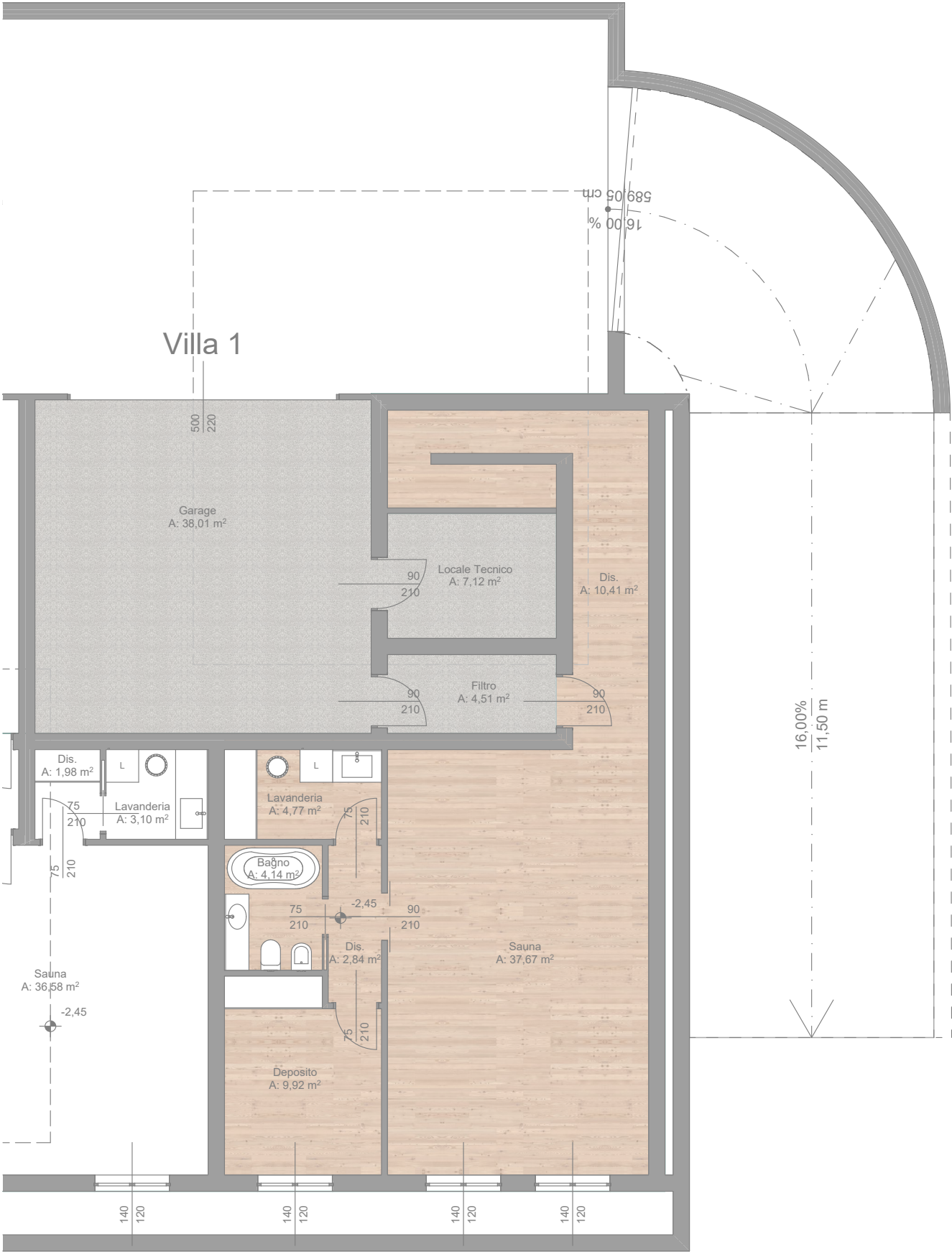
PI Villa_1 1:100
