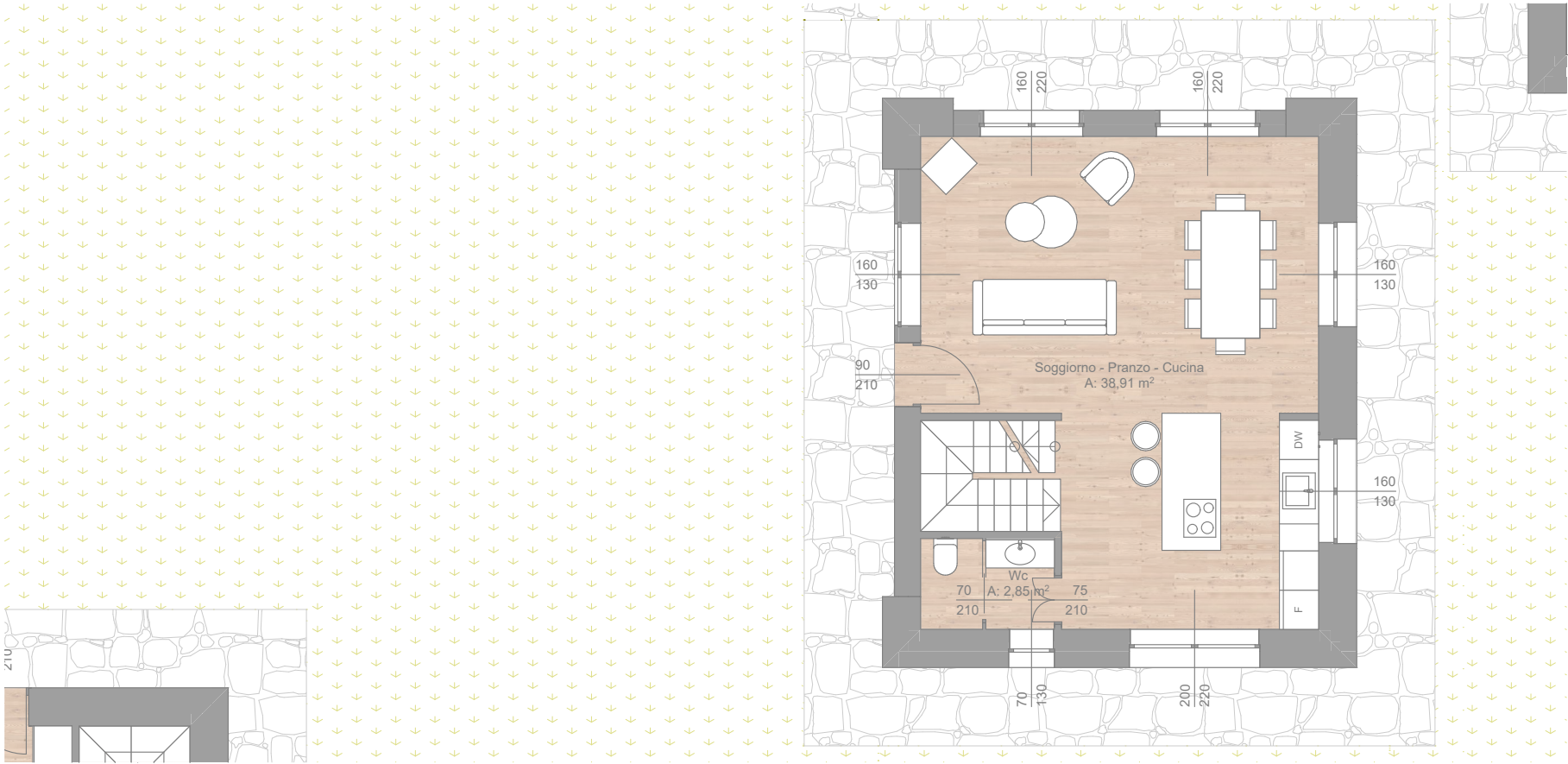
PT Villa_2 1:100
