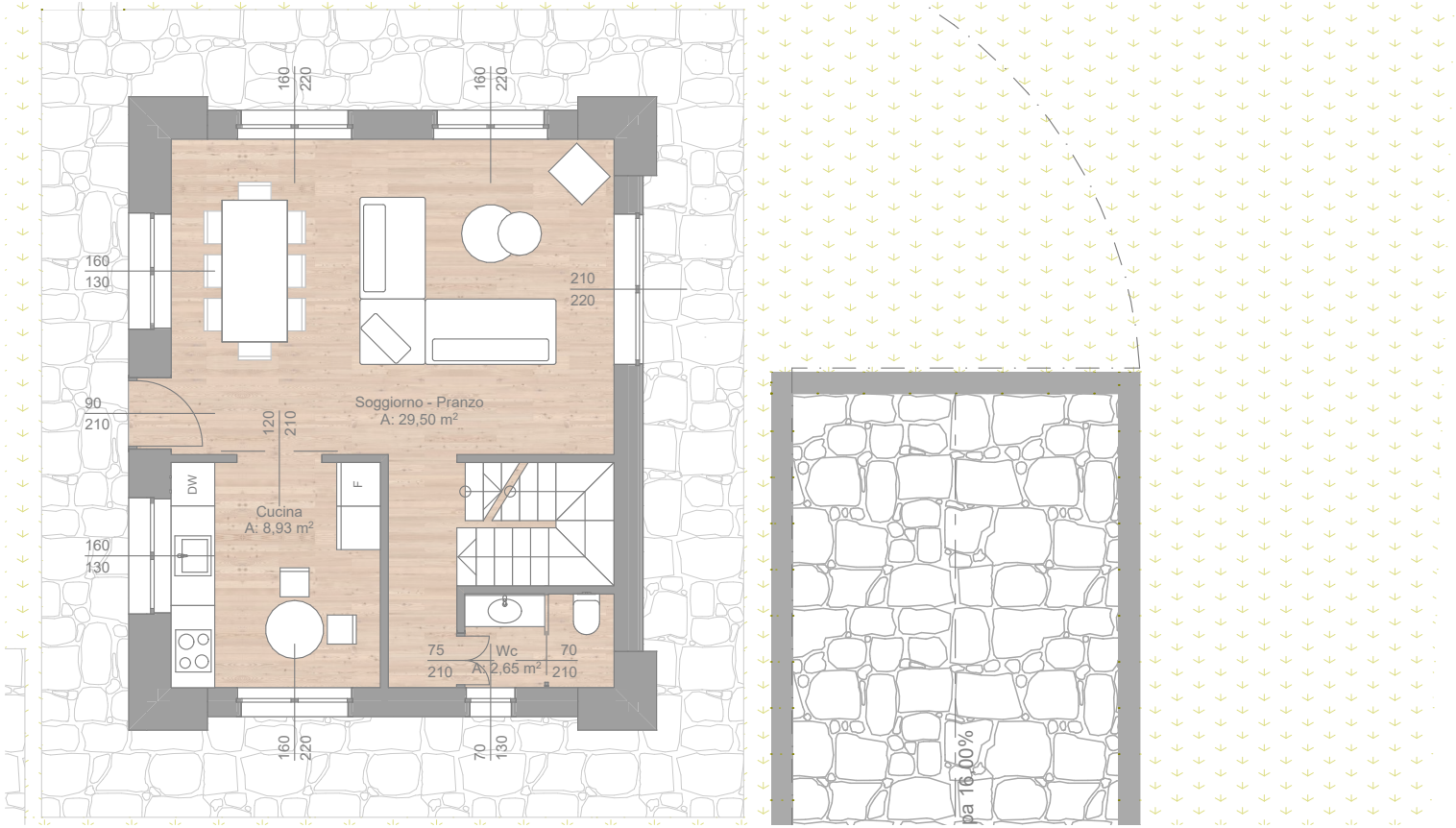
PT Villa_1 1:100
