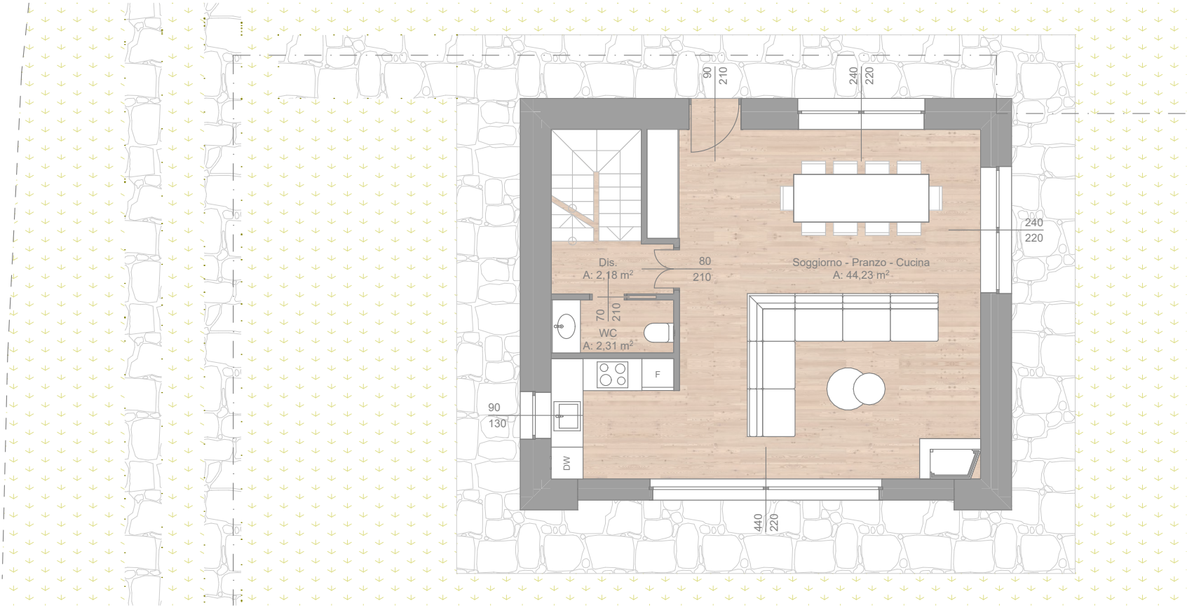
PT Villa_3 1:100
