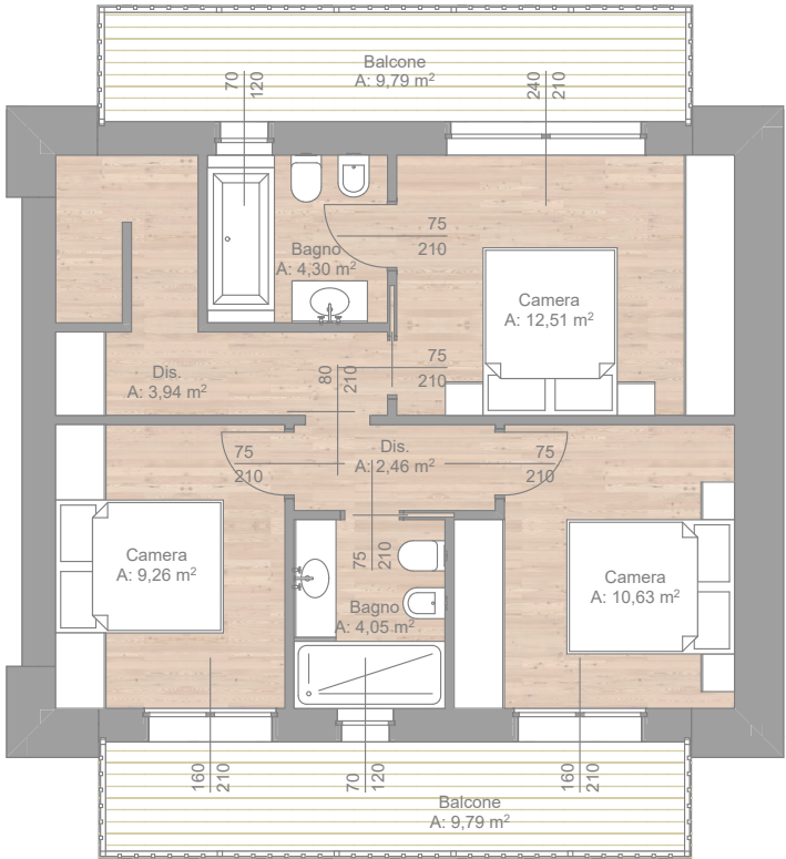
P1 Villa_3 1:100
